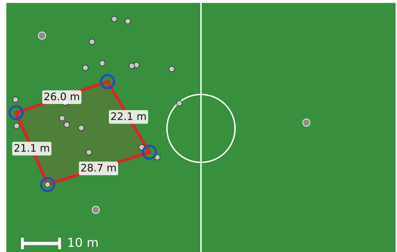
(d) Tactical H_1 ( \delta = 11.75 m)
